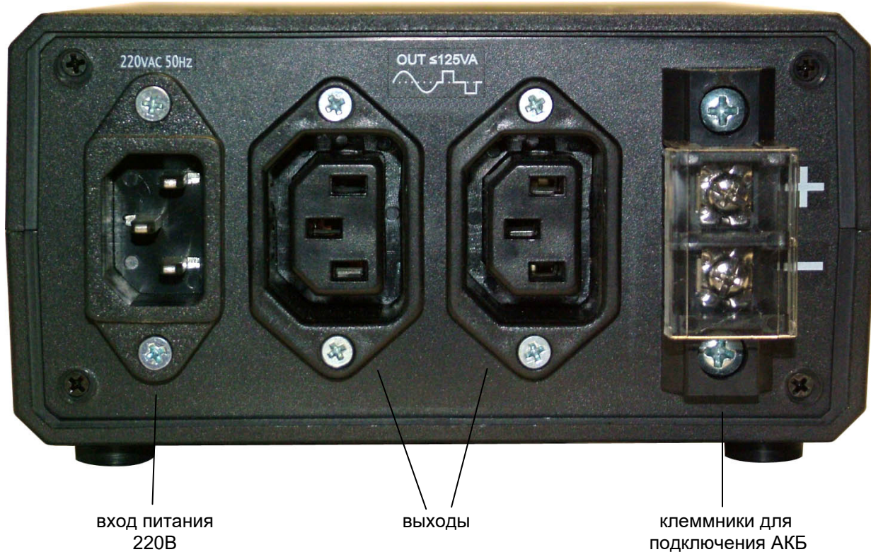
Рис. 2 Задняя панель
