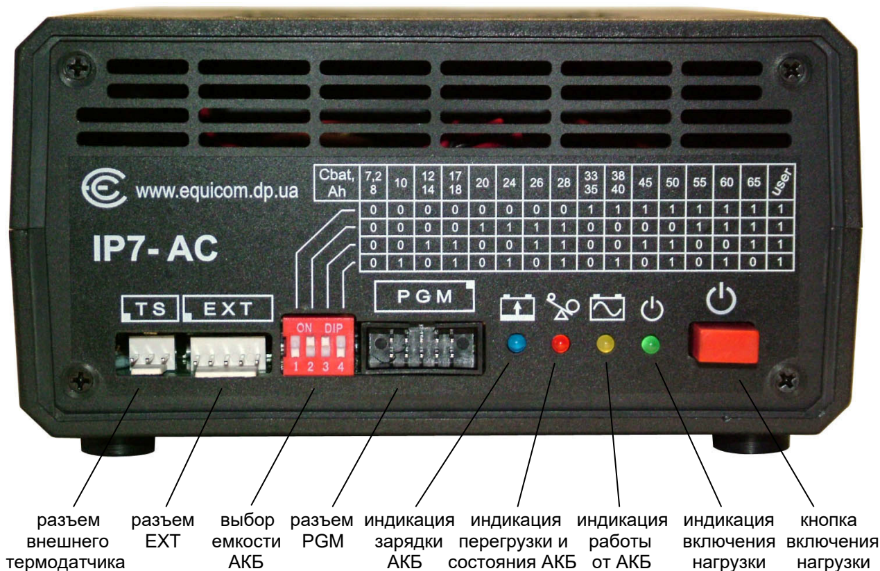
Рис. 1 Передняя панель
