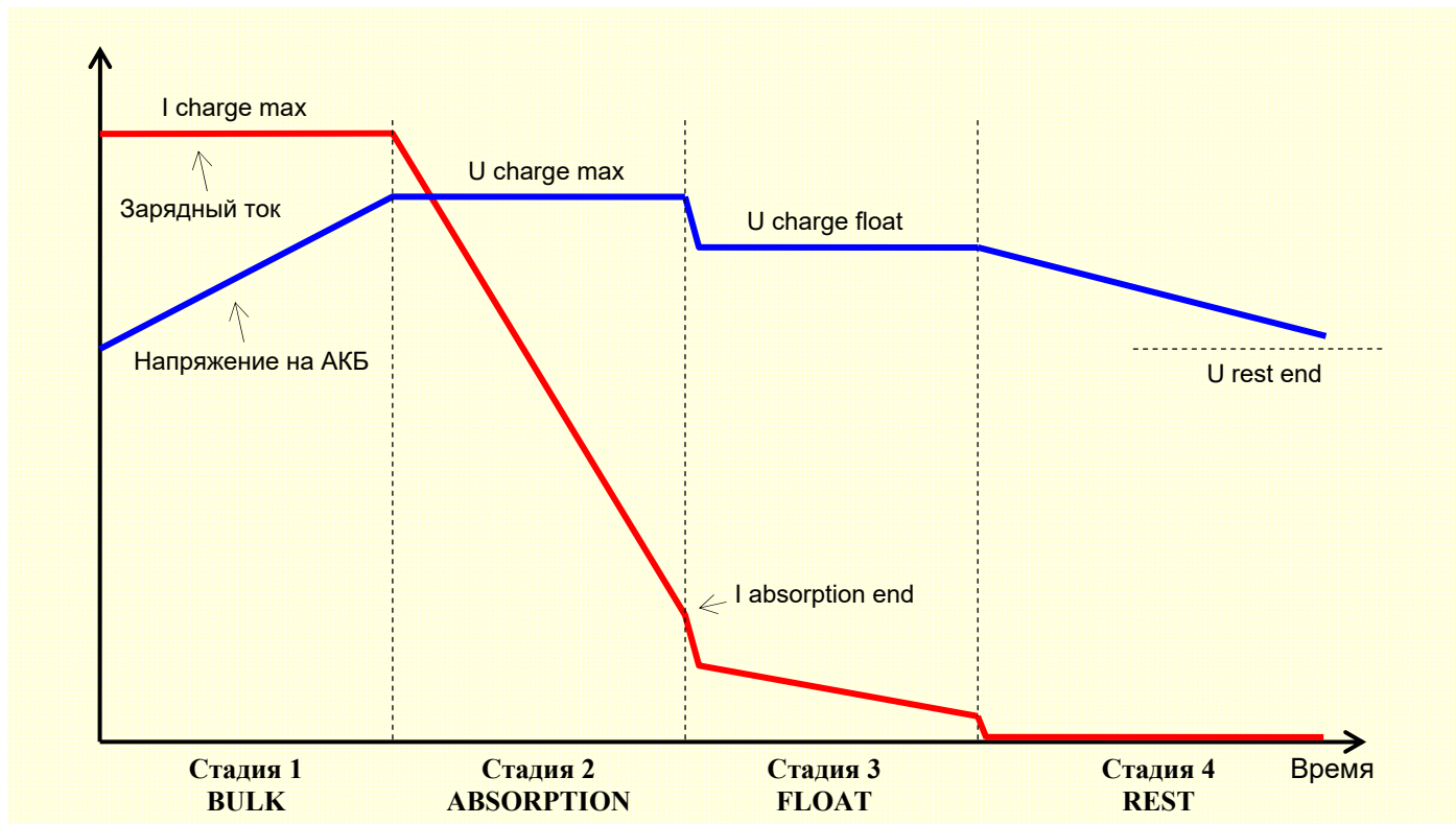
Рис. 8 Стадии четырехступенчатой зарядки АКБ
